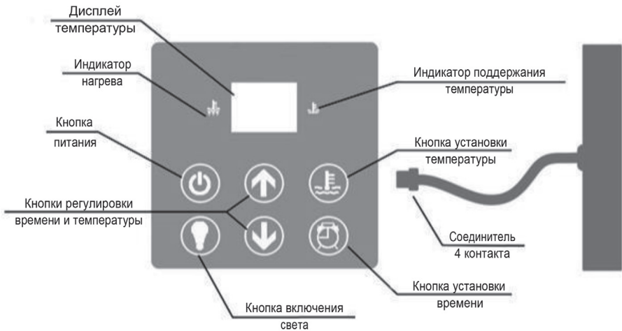
Рисунок 3. Панель управления
