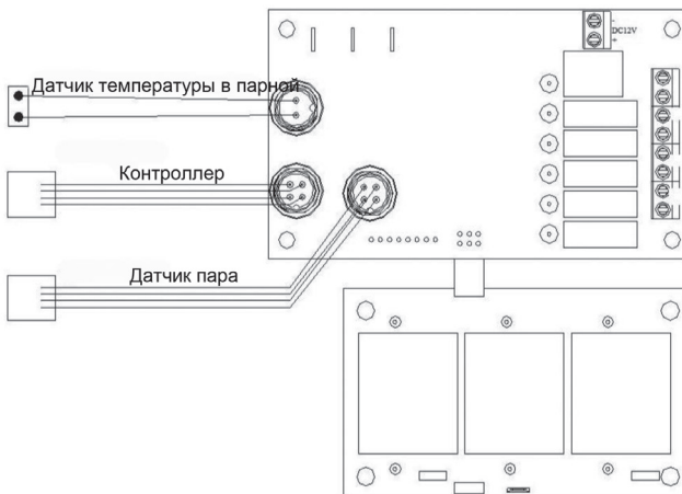
Рисунок 8. Схема подключения электропитания
