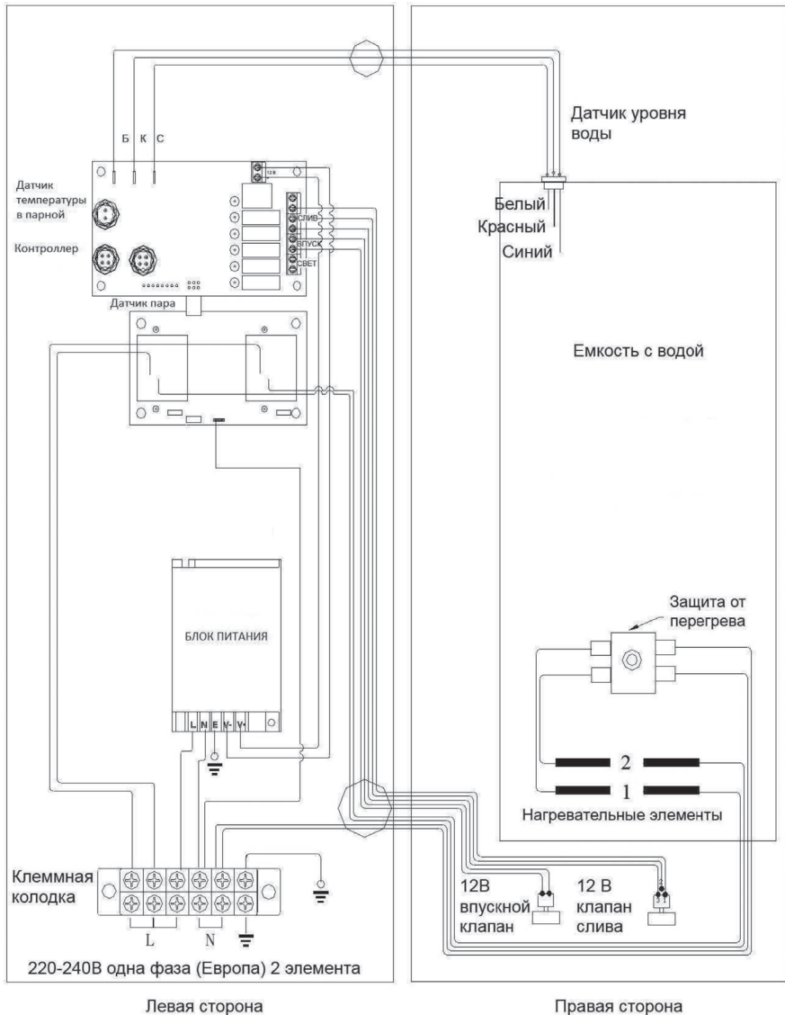
Рисунок 9. Электромонтажная схема TOLO-30 KEY
