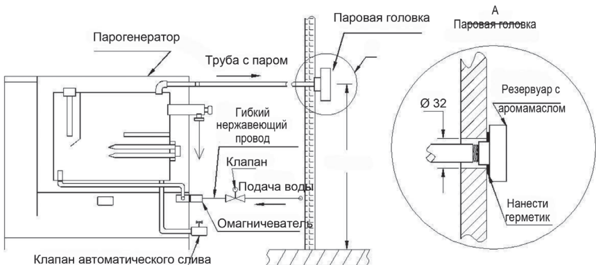
Рисунок 7. Схема установки труб
