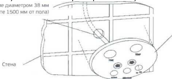
Рисунок 4. Схема установки контроллера на стену
